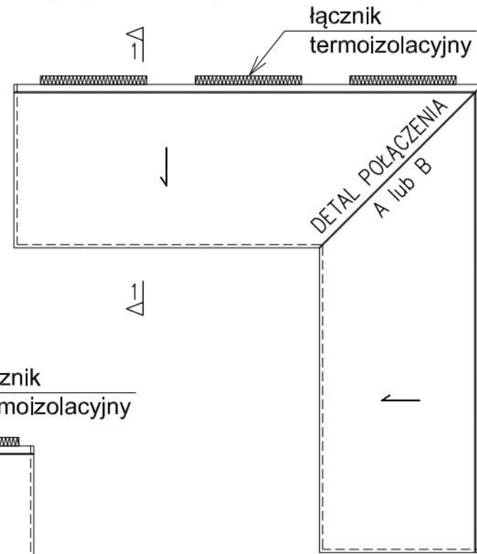
BALKON narożny wewnętrzny (sposób podziału 1)
