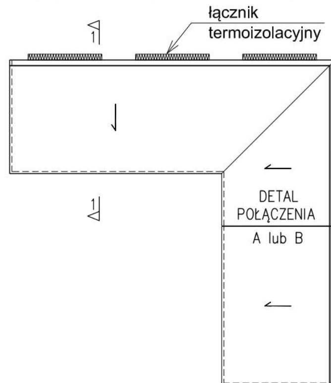
BALKON narożny wewnętrzny (sposób podziału 2)
