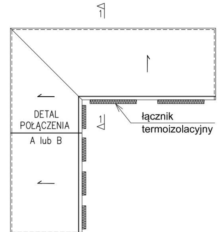
BALKON narożny zewnętrzny (sposób podziału 2)
