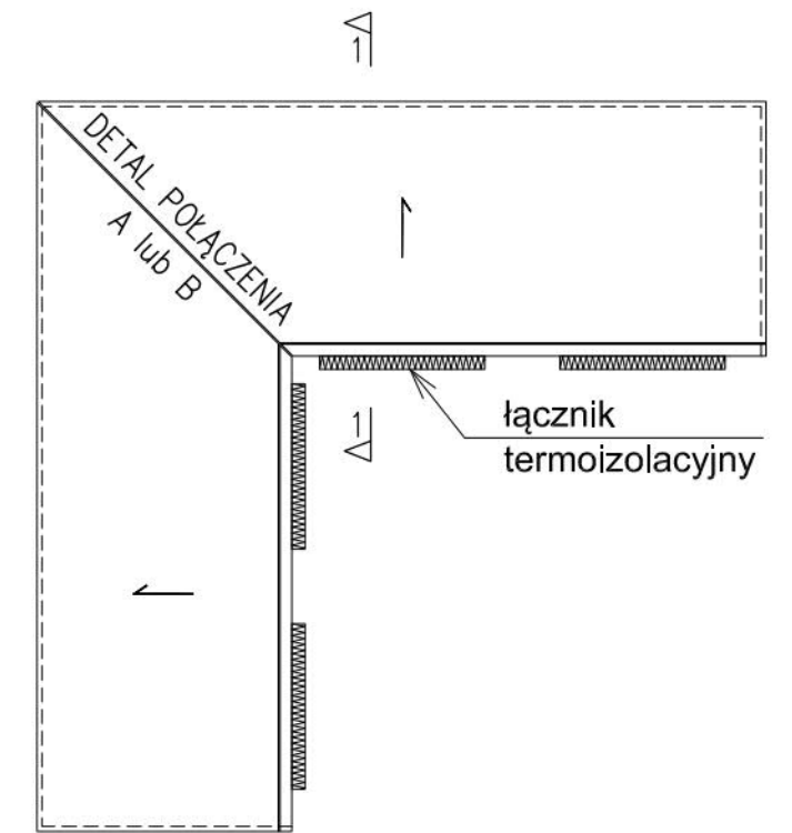
BALKON narożny zewnętrzny (sposób podziału 1)
