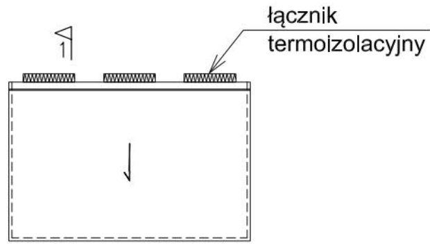
BALKON wspornikowy galeriowy
