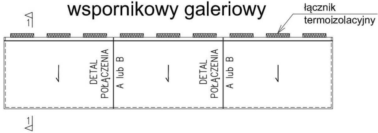
DETAL A
